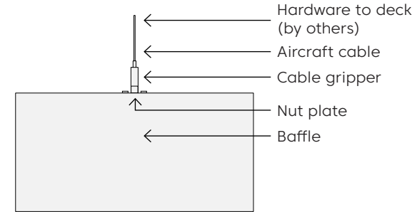
Cable
